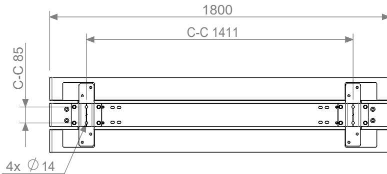
4003A - Dimensions
